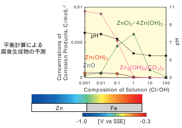
溶液中で Zn と Fe の間に生じる電位分布の計算例
